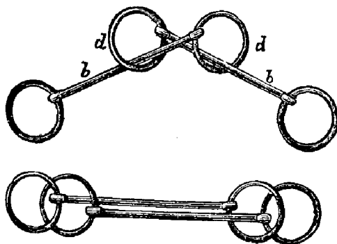
Рис. 389. Предохранительныя удила.
