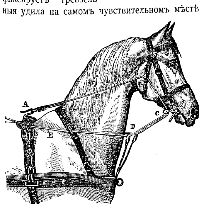
Рис. 403. Американскій усовершенствованный оберъ-чекъ, дѣйствующій какъ шлифцигель.
